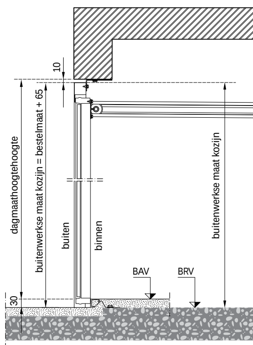
Verticale doorsnede
