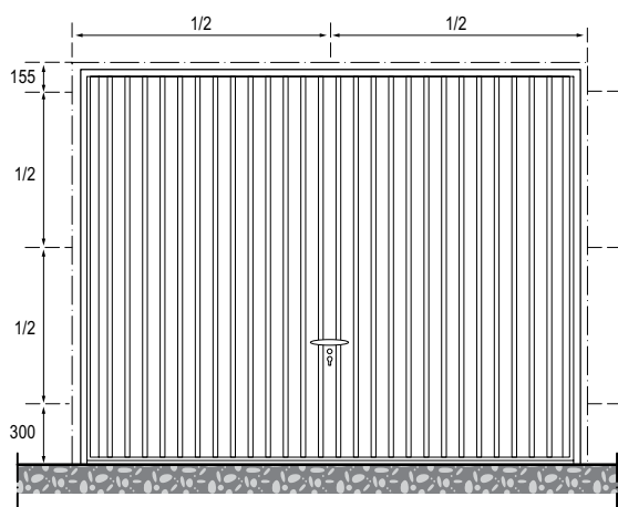
Vooraanzicht met ankeropstelling
