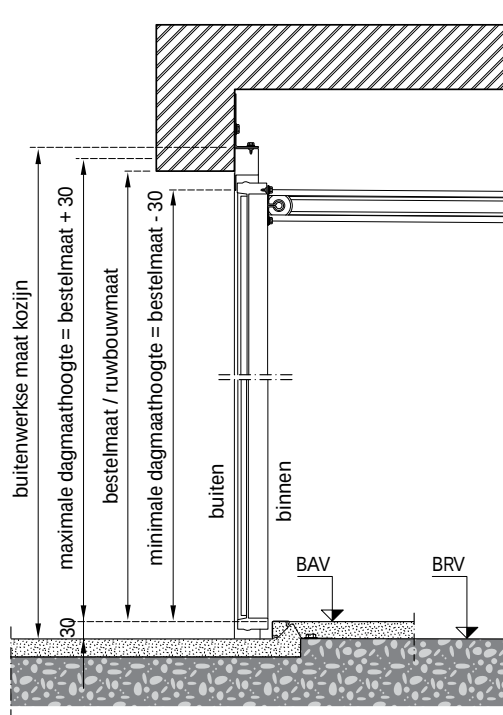
Verticale doorsnede
