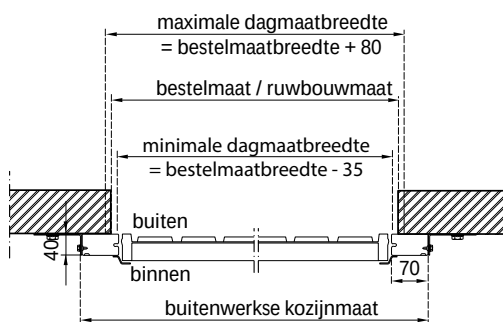
Horizontale doorsnede
