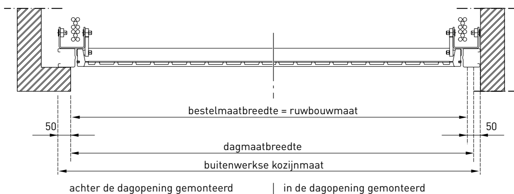
horizontale doorsnede
