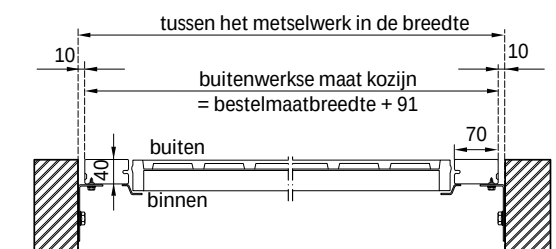
Horizontale doorsnede
