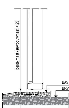
Detail A: zonder aanslag
