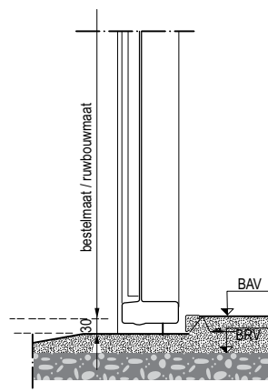
Detail B: met aanslag
